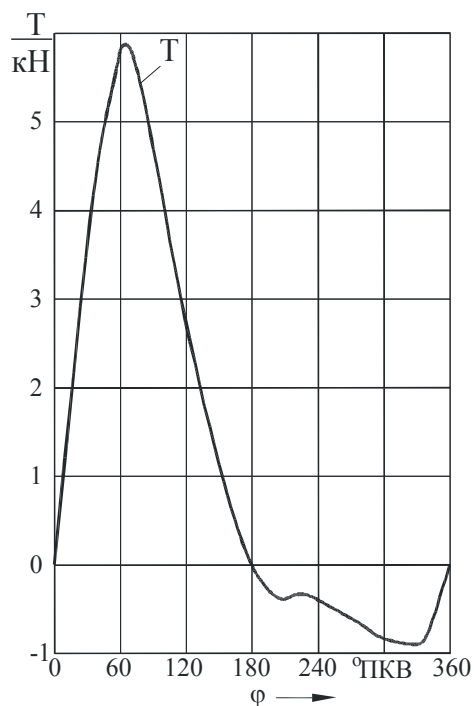
Рис. 6. Изменение по углу поворота кривошипа \varphi тангенциальной силы T на номинальном режиме работы пневмодвигателя (20 кВт, 923 мин -1 )
