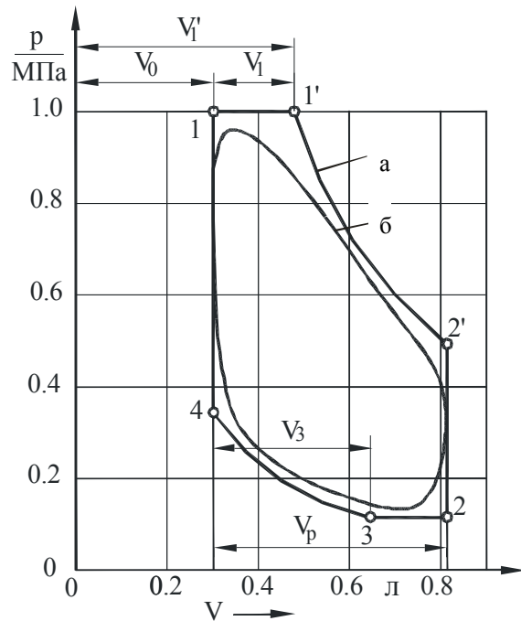
Рис. 3. Расчетные теоретическая (а) и действительная (б) индикаторные диаграммы исследуемого пневмодвигателя: V_p – рабочий объем; V_0 – мертвый объем; V_1 – объем наполнения; V_3 – объем обратного сжатия
