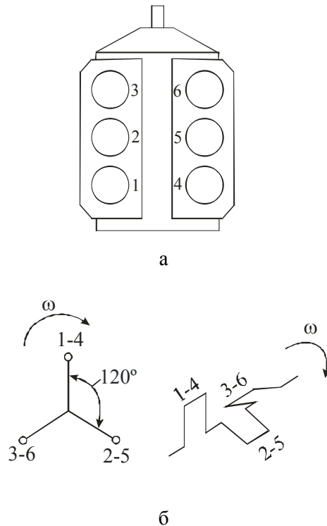
Рис. 1. Схема 6-цилиндрового V-образного пневмодвигателя: а – общая схема двигателя с указанием нумерации цилиндров; б – расположение кривошипов коленчатого вала
