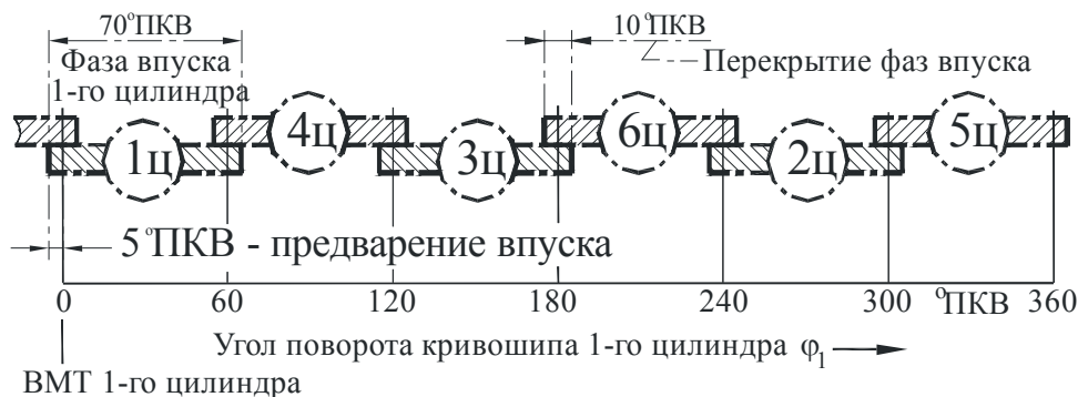
Рис. 2. Принятое в результате выполненного исследования расположение фаз впуска сжатого воздуха в пневмодвигателе
