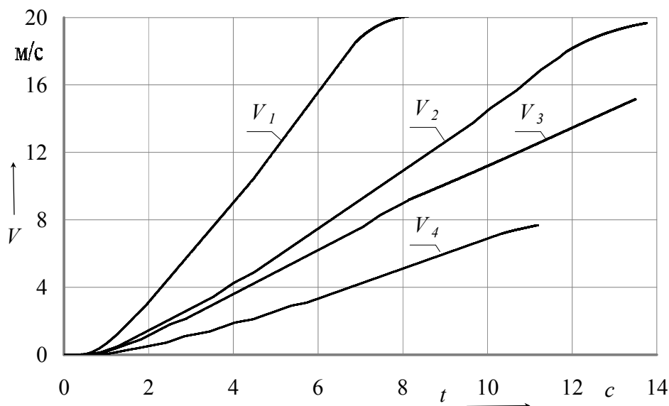
Рис. 8 Залежність швидкості руху транспортного засобу від часу при різних темпах натисканнях на педаль газу
