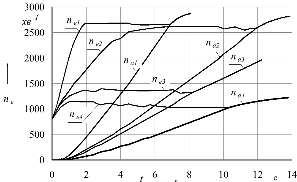
Рис. 7 Зміна частоти обертання колінчатого валу та первинного валу коробки передач в залежності від часу при різних темпах натисканнях на педаль газу
