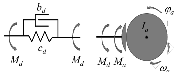
Рис. 4 Розрахункова схема для визначення кута повороту первинного валу ступеневої коробки передач
