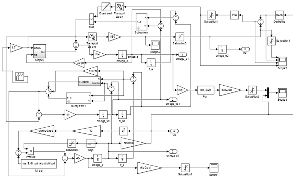
Рис. 6 Реалізація математичної моделі рухання автомобіля з місця у середовищі Simulink пакету MATLAB
