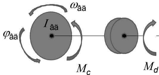
Рис. 3 Розрахункова схема деталей зчеплення, що обертаються
