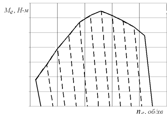
Рис. 2 Залежність моменту двигуна від частоти обертання його колінчатого валу та положення педалі подачі палива
