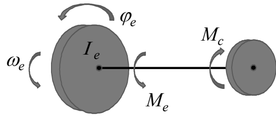
Рис. 1 Розрахункова схема деталей двигуна, що обертаються
