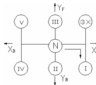
Рис. 2. Траєкторія переміщення МПП при перемикачів з «нейтралі» на першу передачу
