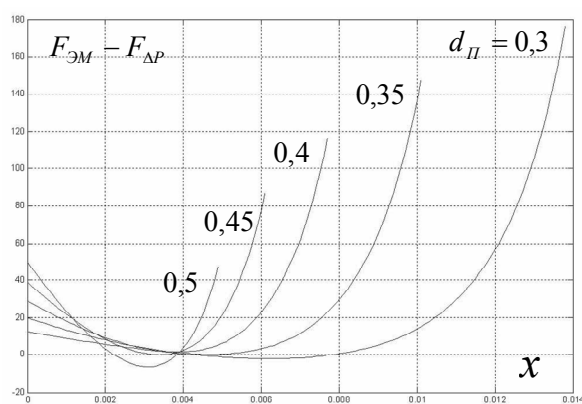
Рис. 6. Результаты оптимизации мощности ЭМ C_{ЭМ}
