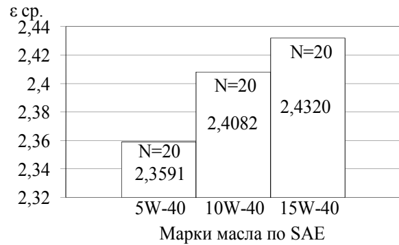
Рис. 2. Средние значения \varepsilon масел различных марок (классов вязкости) по SAE
