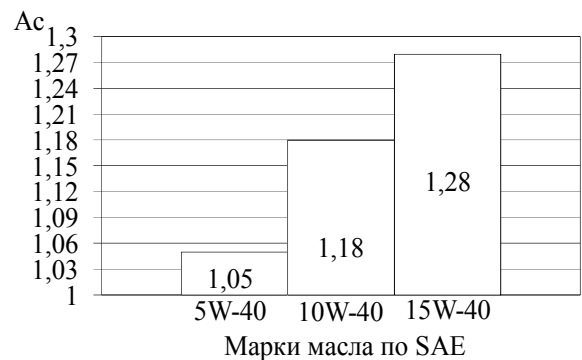
Рис. 3. Средние значения сульфатной золы для масел различных марок (классов вязкости) по SAE
