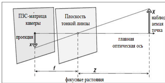
Рис. 2. Модель видеокамеры
