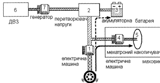
Гальмівне зусилля
