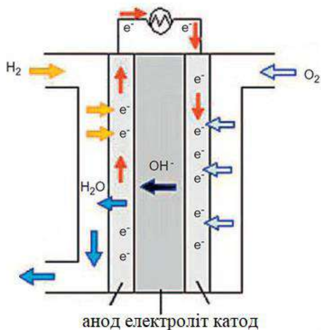
Рис. 8.13. Воднево-кисневий паливний елемент
