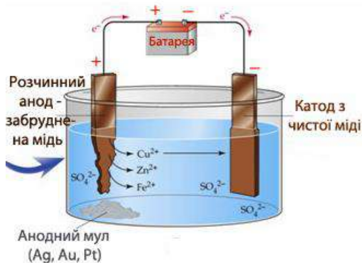
Рис. 8.35. Електрорафінування міді
