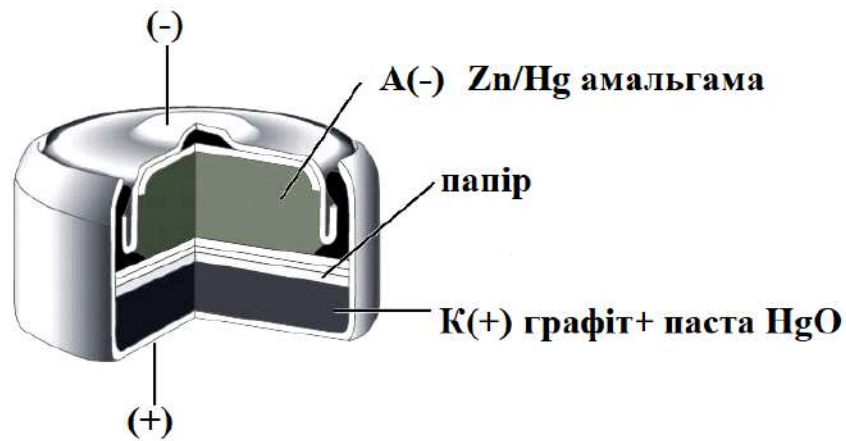
Рис. 8.7. Окисно-ртутний елемент
