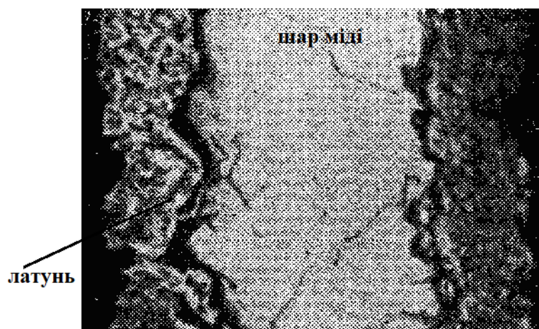
Рис. 8.17. Знецинкування латуні
