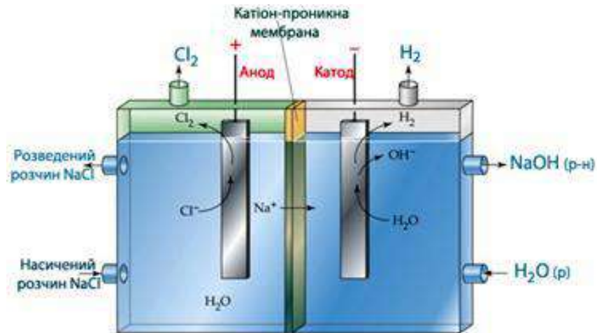
Рис. 8.36. Отримання гідроксиду натрію та хлору
