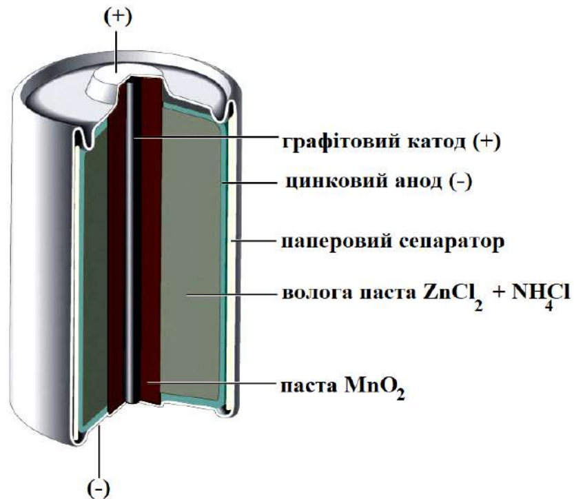
Рис. 8.6. Марганцево-цинковий елемент (елемент Лекланше)
