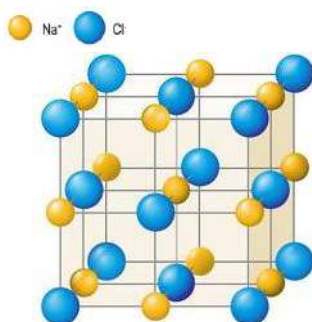
Рис. 3.1. Структура кристалу NaCl
