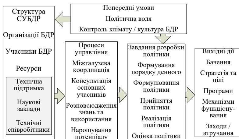
Рис. 5. Принципова схема управління безпекою дорожнього руху
