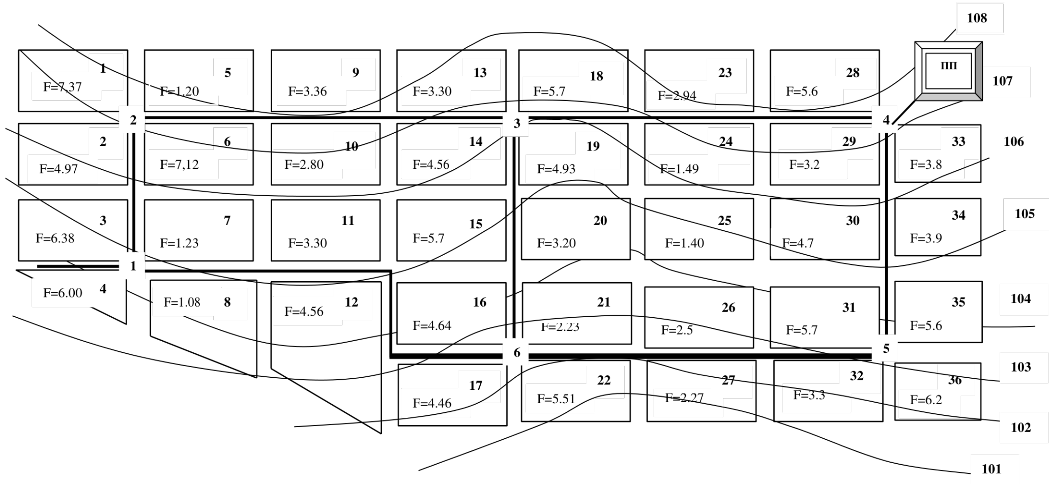
Рисунок 1 – План міста з горизонталями з нанесенням магістральних водогінних мереж
