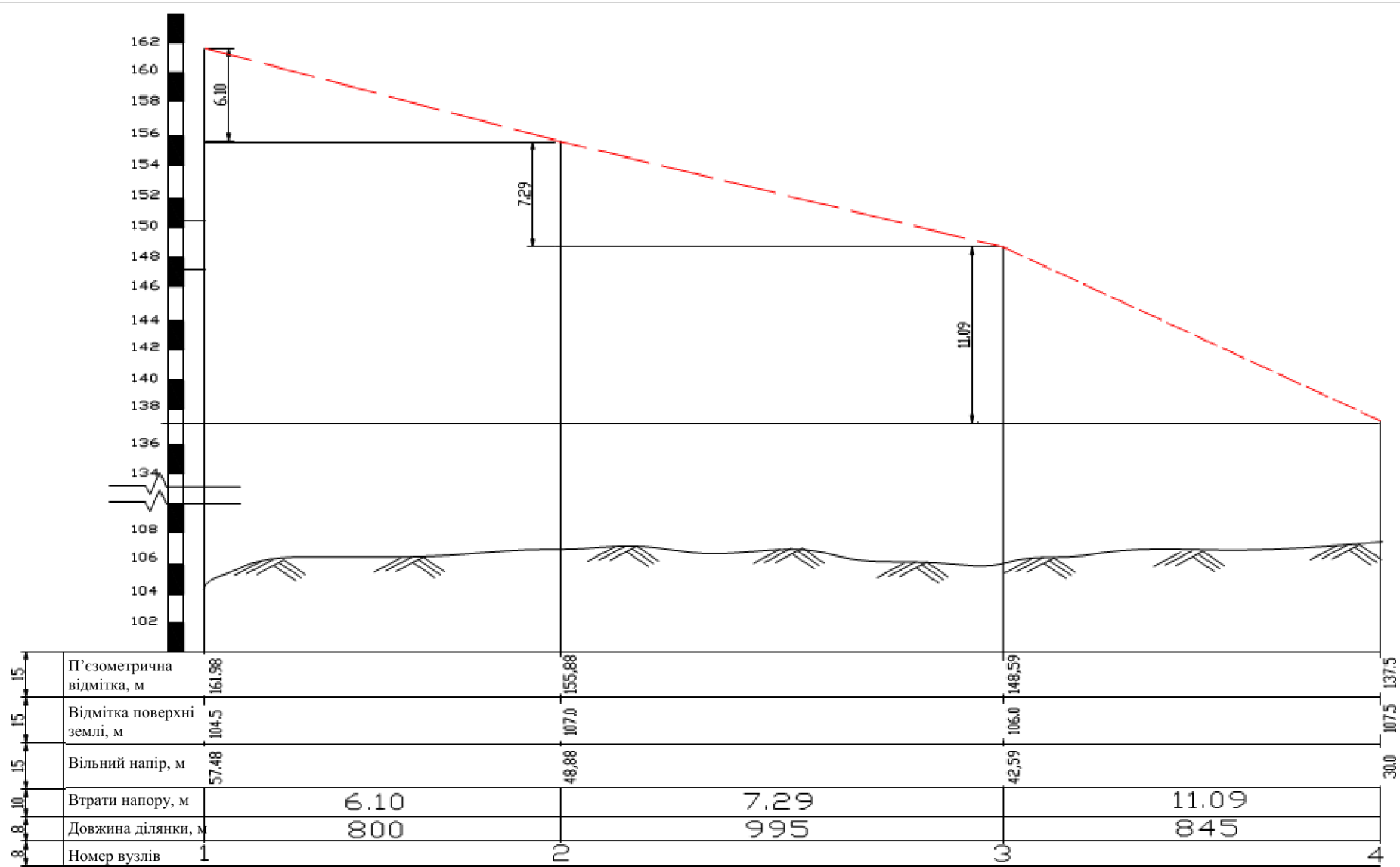
Рисунок 3 – Лінія п'єзометричного тиску
