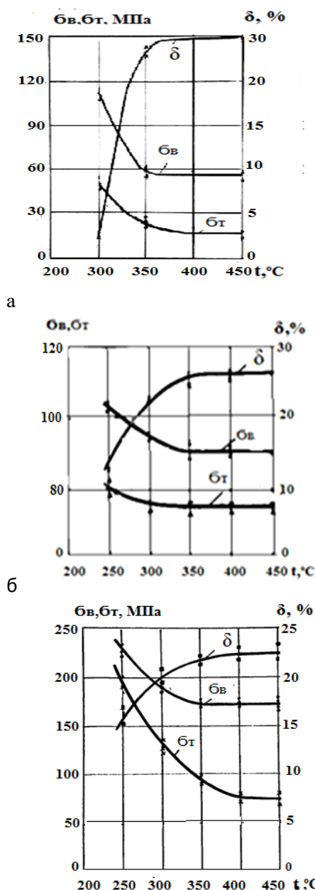
Рис. 1. Залежність механічних властивостей сплавів АД1 (а), АМц (б) АМг3(в) від температури нагріву під час відпалу
