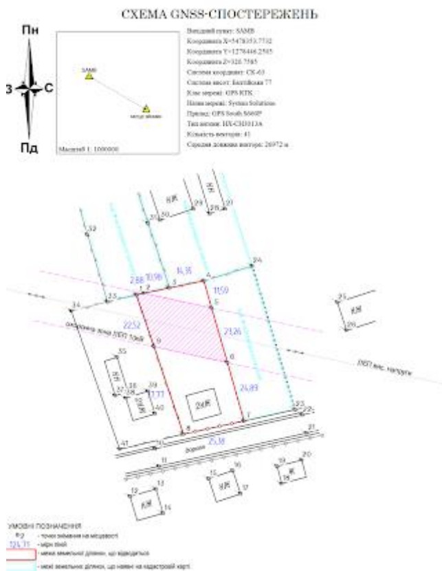
Рис. 2. Схема GNSS-спостережень
