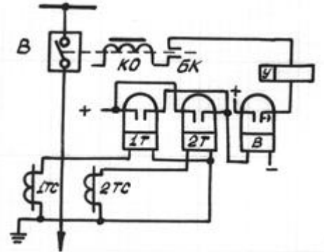
Рисунок – 2 Схема двофазного МСЗ з характеристикою часу спрацьовування на постійному оперативному струмі.
