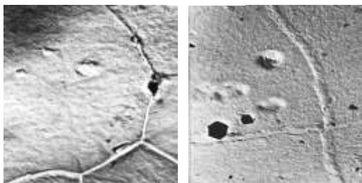
Рис. 5. Мікроструктура сталі 08 кп після відпалу за 700 °С з витримкою 15 с та деформаційного старіння протягом 5 діб (а) і місяця (б); \times 10000
