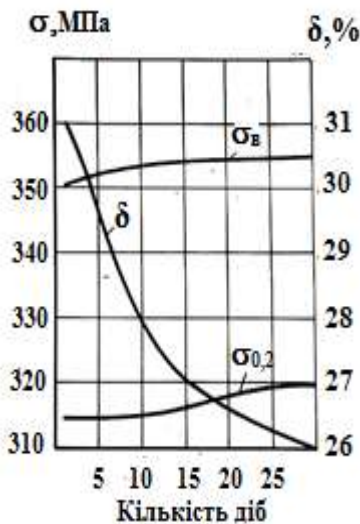
Рис. 8. Механічні властивості сталі 08 кп після відпалу за 700 °С, (витримка 15 с), перестарювання (витримка 30 с) та природного старіння
