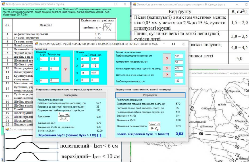
Рис. 2 – Інтерфейс блоку розрахунку на морозостійкість та довідкові вікна
