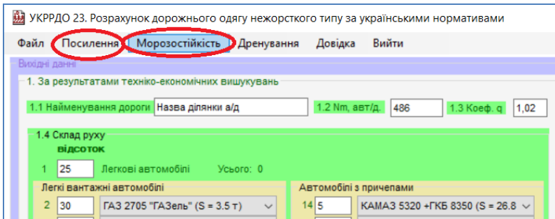
Рис. 2 – Інтерфейс блоку розрахунку на морозостійкість та довідкові вікна
