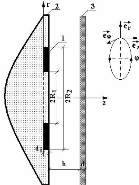
Рис. 1. Расчётная модель
