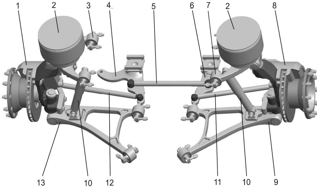
Рис. 1. Підвіска керованих коліс автобуса Богдан А70132: 1 – колісний механізм лівий; 2 – рукавний пружний елемент; 3 – важіль верхній лівий; 4 – важіль кермової трапеції лівий; 5 – тяга кермова поперечна; 6 – важіль кермової трапеції правий; 7 – важіль верхній правий; 8 – колісний механізм правий; 9 – важіль нижній правий; 10 – амортизатор; 11 – тяга кермова права; 12 – тяга кермова ліва; 13 – важіль нижній лівий
