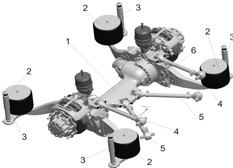
Рис. 2. Підвіска ведучої осі автобуса Богдан А70132: 1 – ведуча вісь; 2 – рукавний пружний елемент; 3 – амортизатор; 4 – верхня реактивна тяга; 5 – нижня реактивна тяга; 6 – зашрубок отвору контролю рівня оливи
