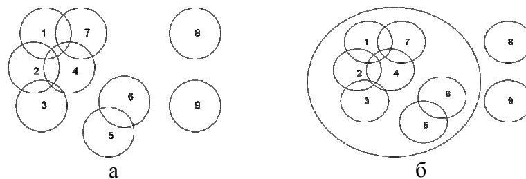
Рис. 1. Діаграми Ейлера-Венна. Знаходження «об'єднаної» множини
