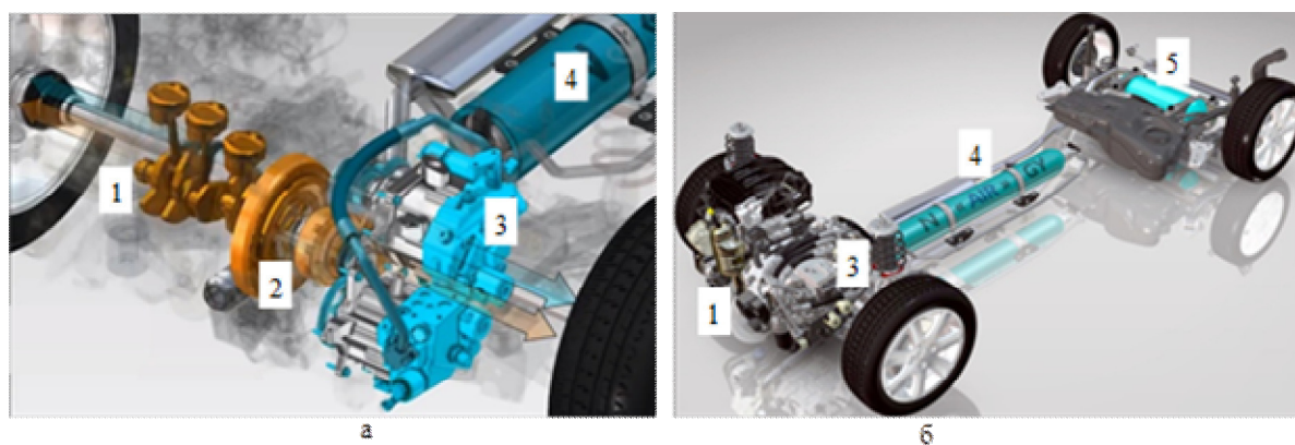
Рис. 2. Гибридная технология Hybrid Air: а – устройство силовой установки; а – компоновка силовых агрегатов на шасси
