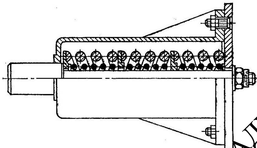
Рисунок 2.2 – Буфер із концентричним набором крутильних циліндричних пружин
